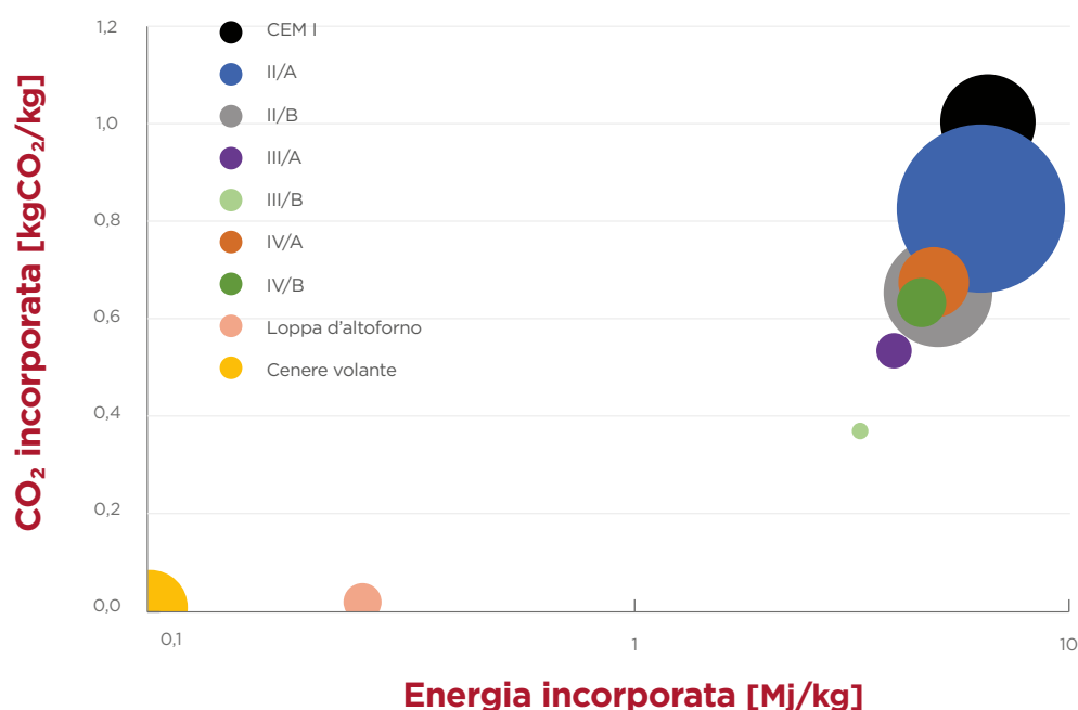
Figura 2 - Energia ed anidride carbonica incorporata in diversi leganti tradizionali e materiali cementizi supplementari. La dimensione del cerchio rappresenta il volume di produzione annuo italiano (per le ceneri volanti si riporta la somma dei tipi V e W). Dati rielaborati da [10,13 e 14]
