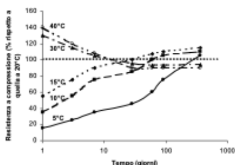
Figura 1 - Resistenza meccanica a compressione in funzione del tempo di calcestruzzi maturati a temperature comprese tra 5°C e 40°C
