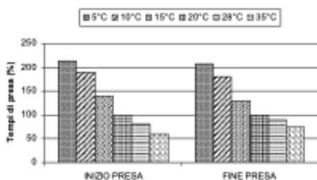
Figura 3 - Tempi di inizio e fine presa del calcestruzzo (CEM II/B-LL 32.5, a/c=0.60) in funzione della temperatura
