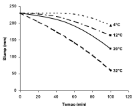
Figura 2 - Lavorabilità del calcestruzzo (CEM II/B-LL 32,5, a/c=0.60 ) in funzione del tempo e della temperatura del conglomerato
