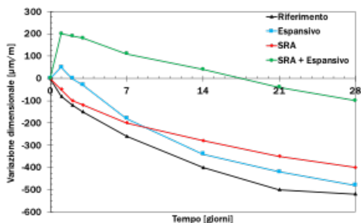
Figura 1 – Espansione/ritiro su provini di calcestruzzo confezionate senza e con SRA e agenti espansivi a base di ossido di calcio esposti all'aria subito dopo il getto.
